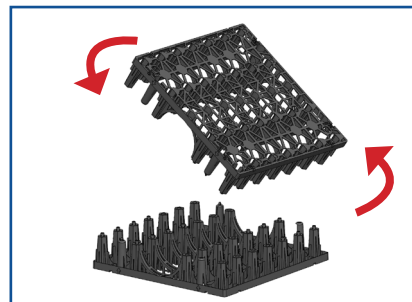
3. Drej øverste element 180°.
